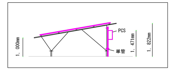
※1 第1柱断面図
