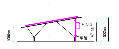
架台 立面図
