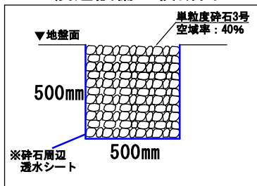
第1柱 断面図
