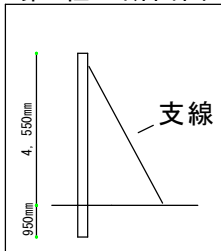
第1柱 断面図
