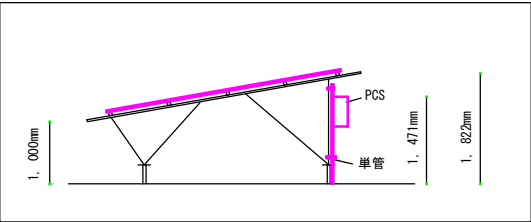
PCS断面図
