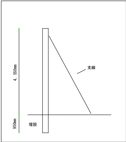
PCS断面図
