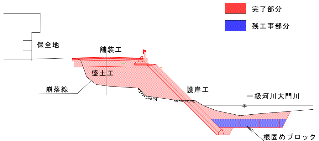
<代表横断図>
