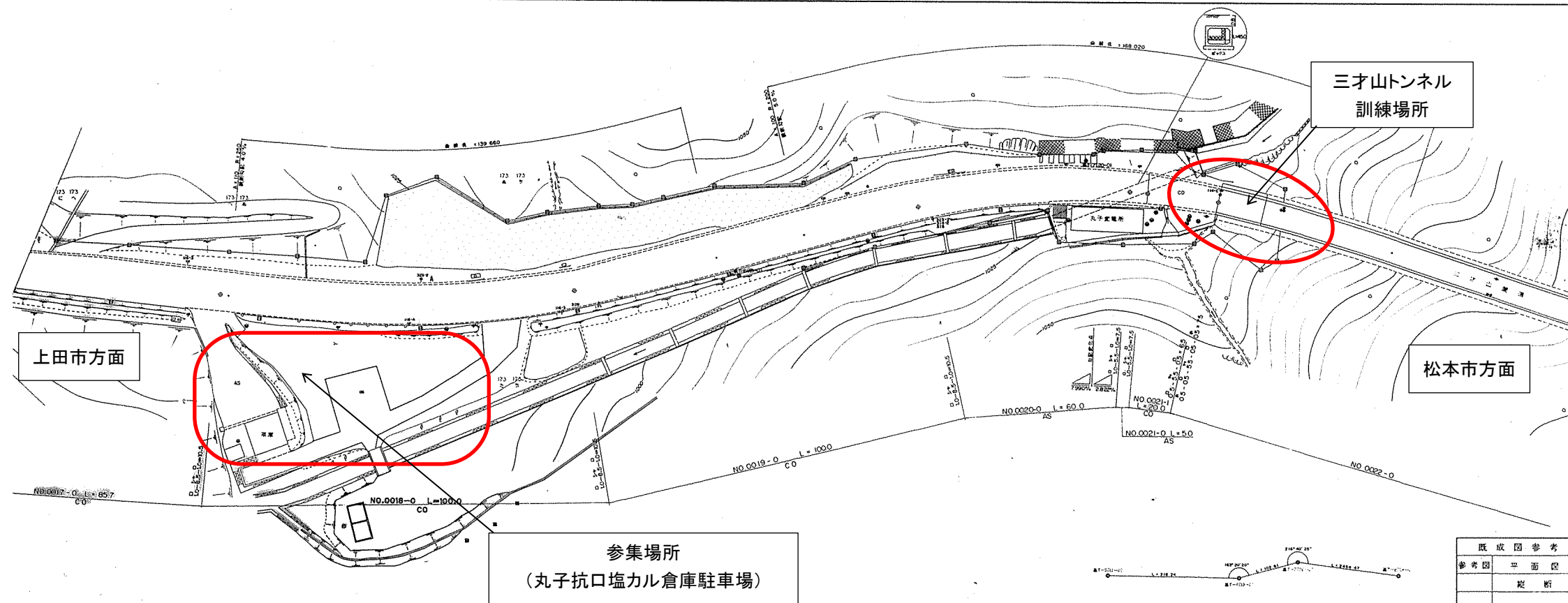
道路台帳平面図 S=1:500 (占用物件図)
