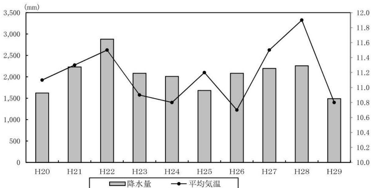
図8-1 気象概況
