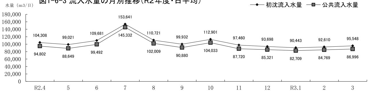
図1-6-3 流入水量の月別推移(R2年度・日平均)
