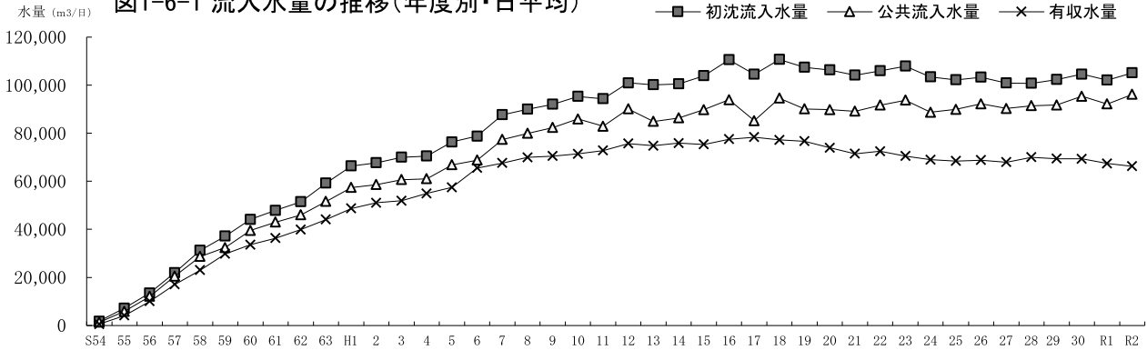
図1-6-1 流入水量の推移(年度別・日平均)
