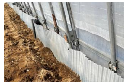
写真10 ハウス内へ波板の埋め込み
