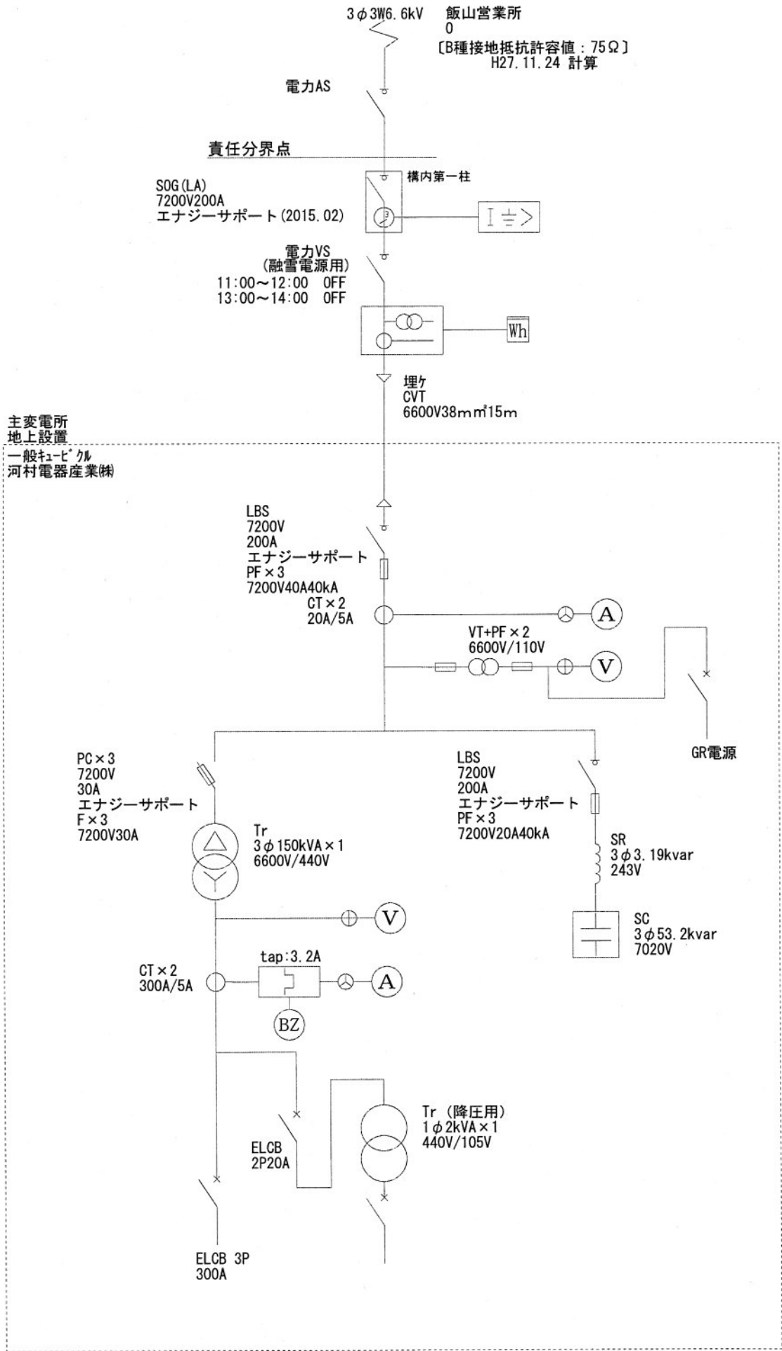
単線結線図 721-7912-1 飯山市大字飯山1140 福寿町無散水融雪施設
