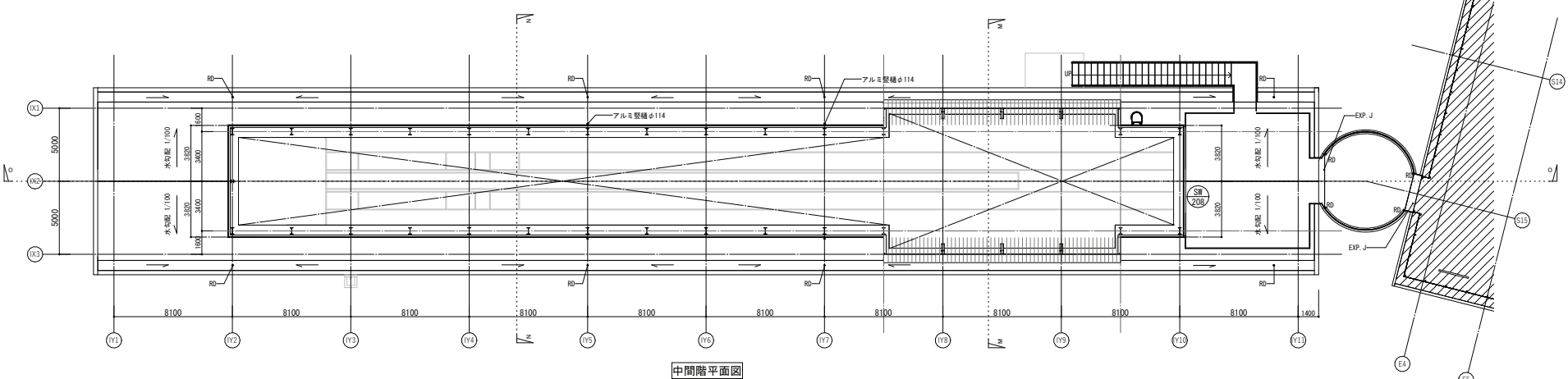
中間階平面図
