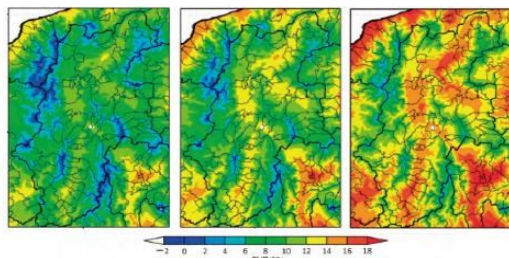
長野県における年平均気温の 将来予測シナリオ：RCP8.5
