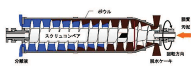
省エネ型遠心脱水機
