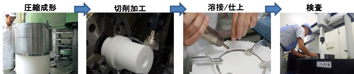
PTFEの製造プロセス
