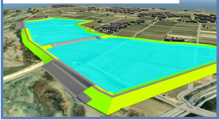
遊水地計画3次元立体モデル図
