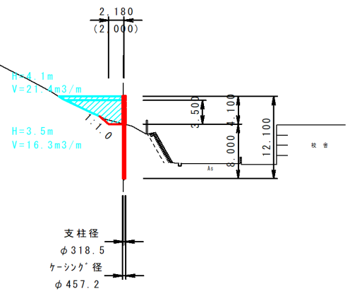
標準横断図
