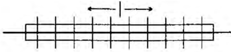
図3-12-1 ボルト締付け順序
