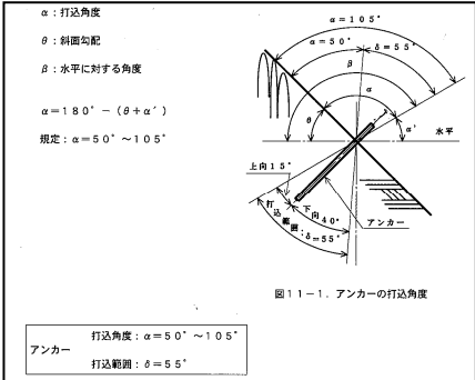
(参考 アンカーの打込角度について)
