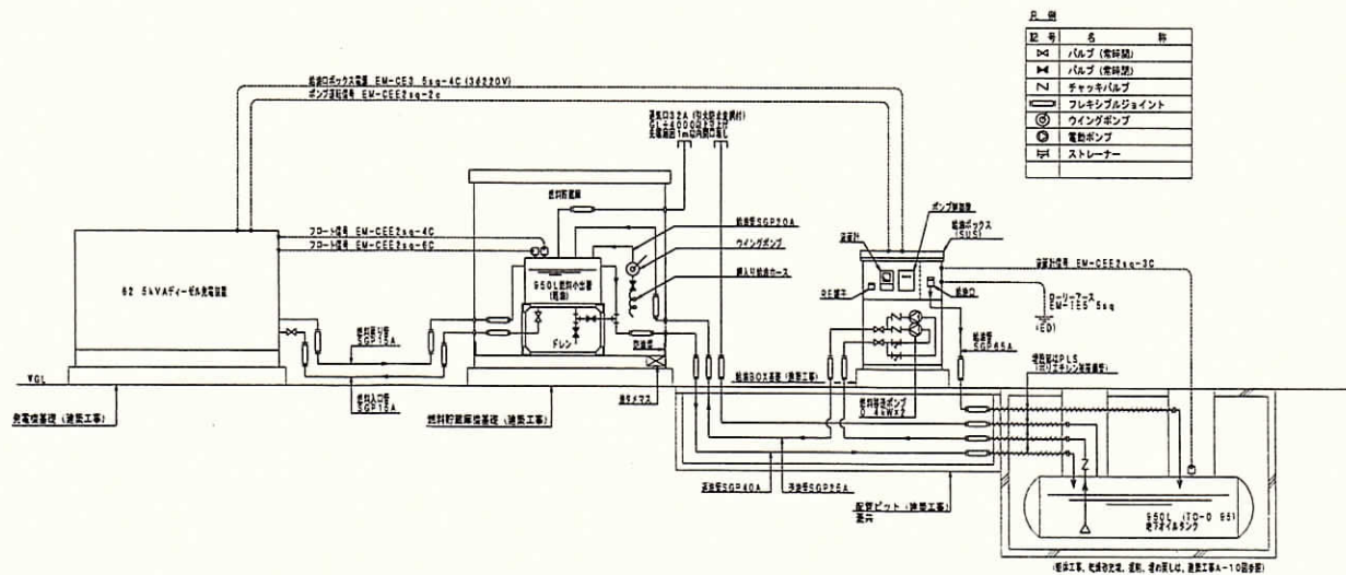
配管系統圖
