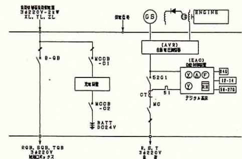
單線結線圖
