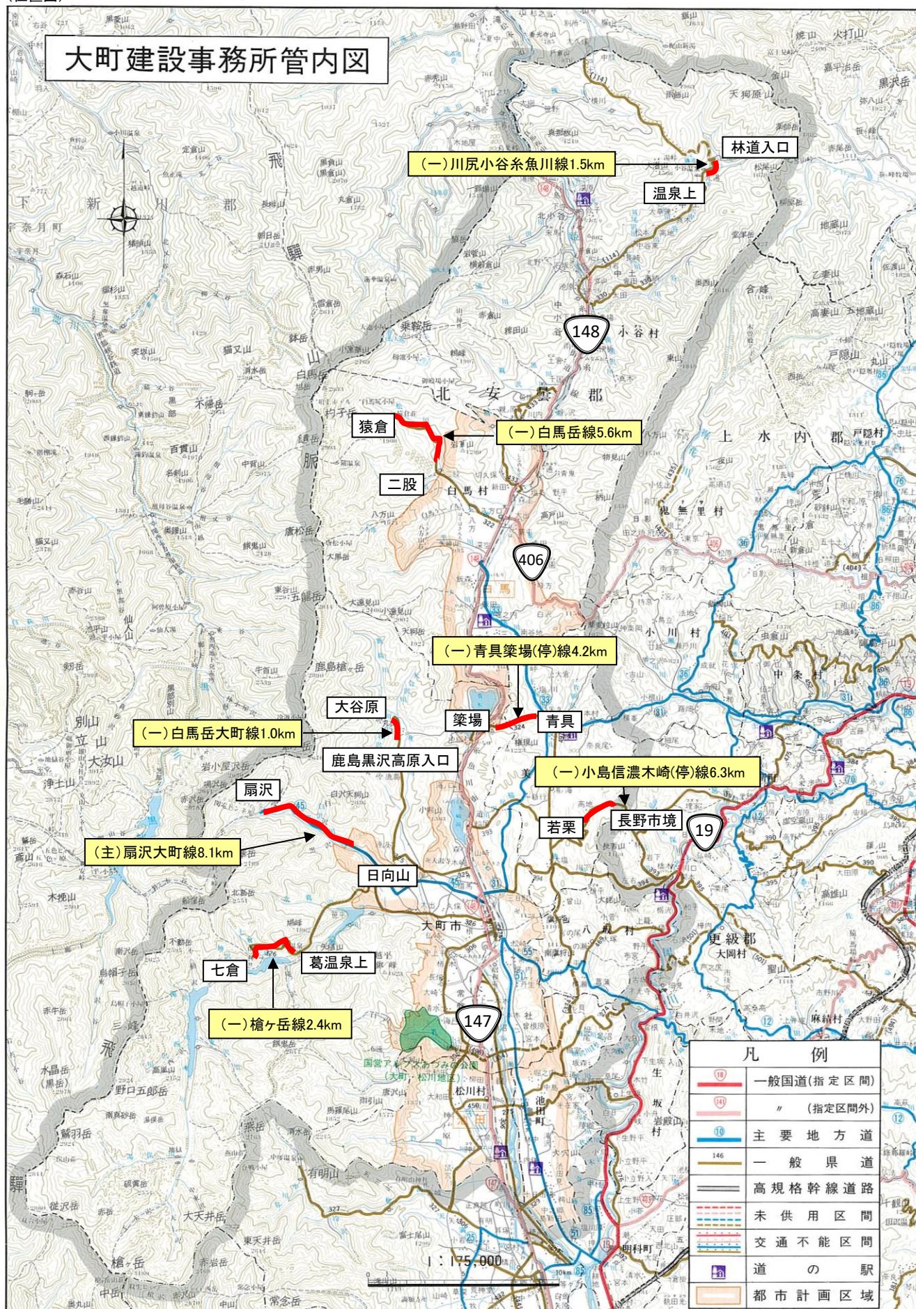
(位置図)
