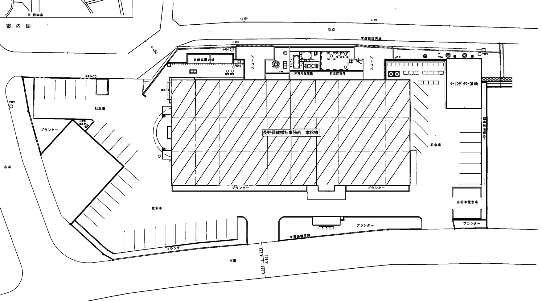
配置図 S=1/200
