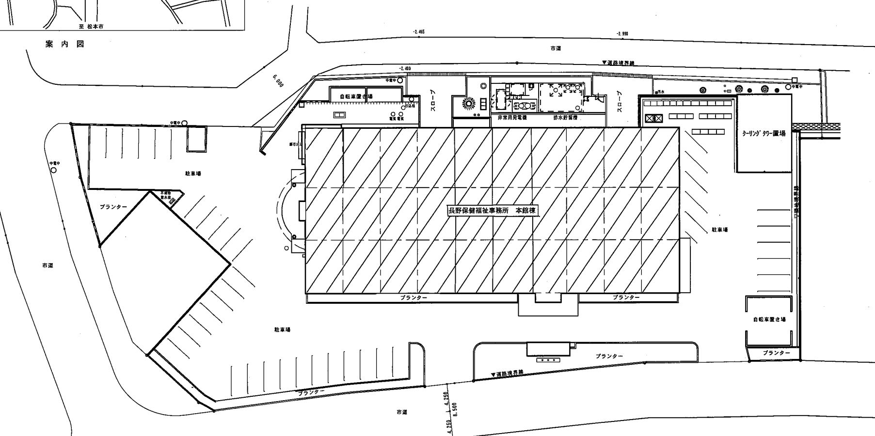
配置図 S=1/200
