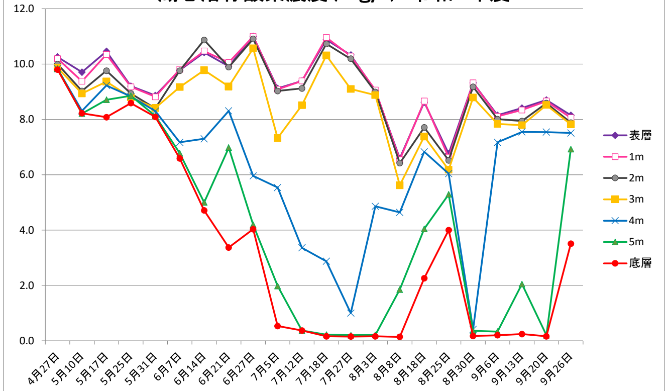
湖心溶存酸素濃度(mg/L):令和5年度
