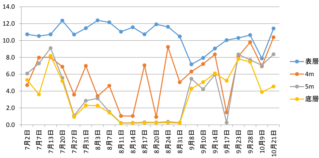
湖心の表層・底層溶存酸素濃度(mg/L):令和2年度
