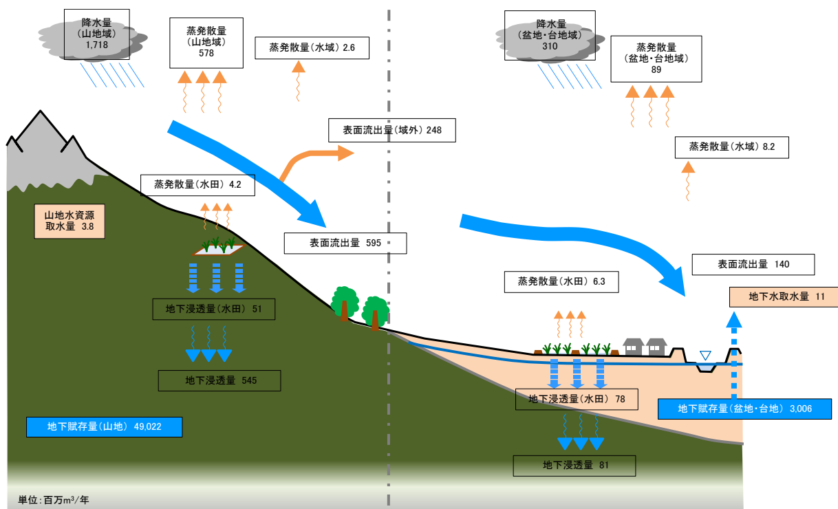
現況の水収支の模式図（北信）
