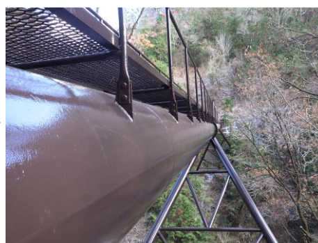
補修が完了した生田寺沢川サイフォン（竜東一貫水路）
