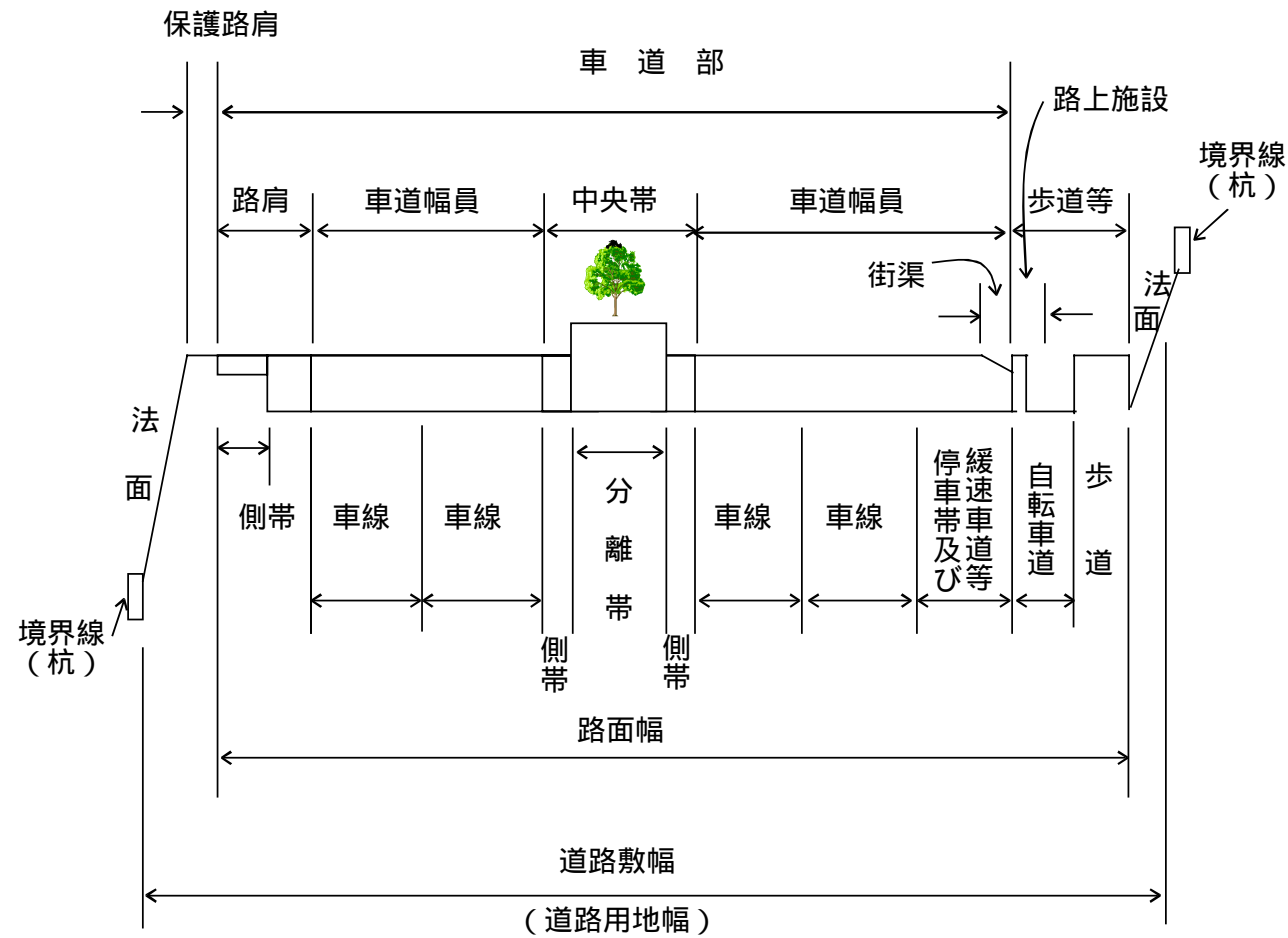
道路の横断面の構成要素
