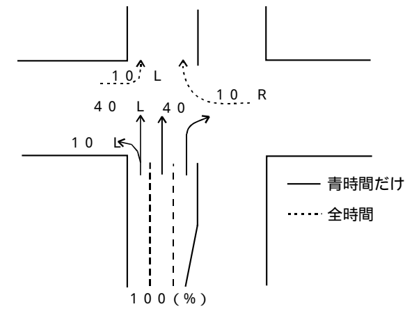
図 右左折車専用車線がある場合の考え方
