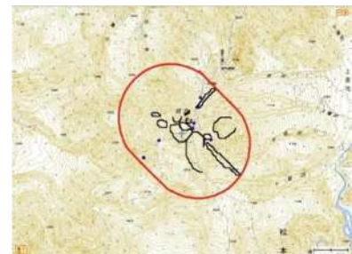
赤線：想定火口 黒線：過去の活動火口 青線：現在の噴気位置
