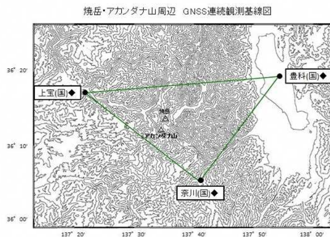
焼岳観測点配置図（国土地理院提供）
