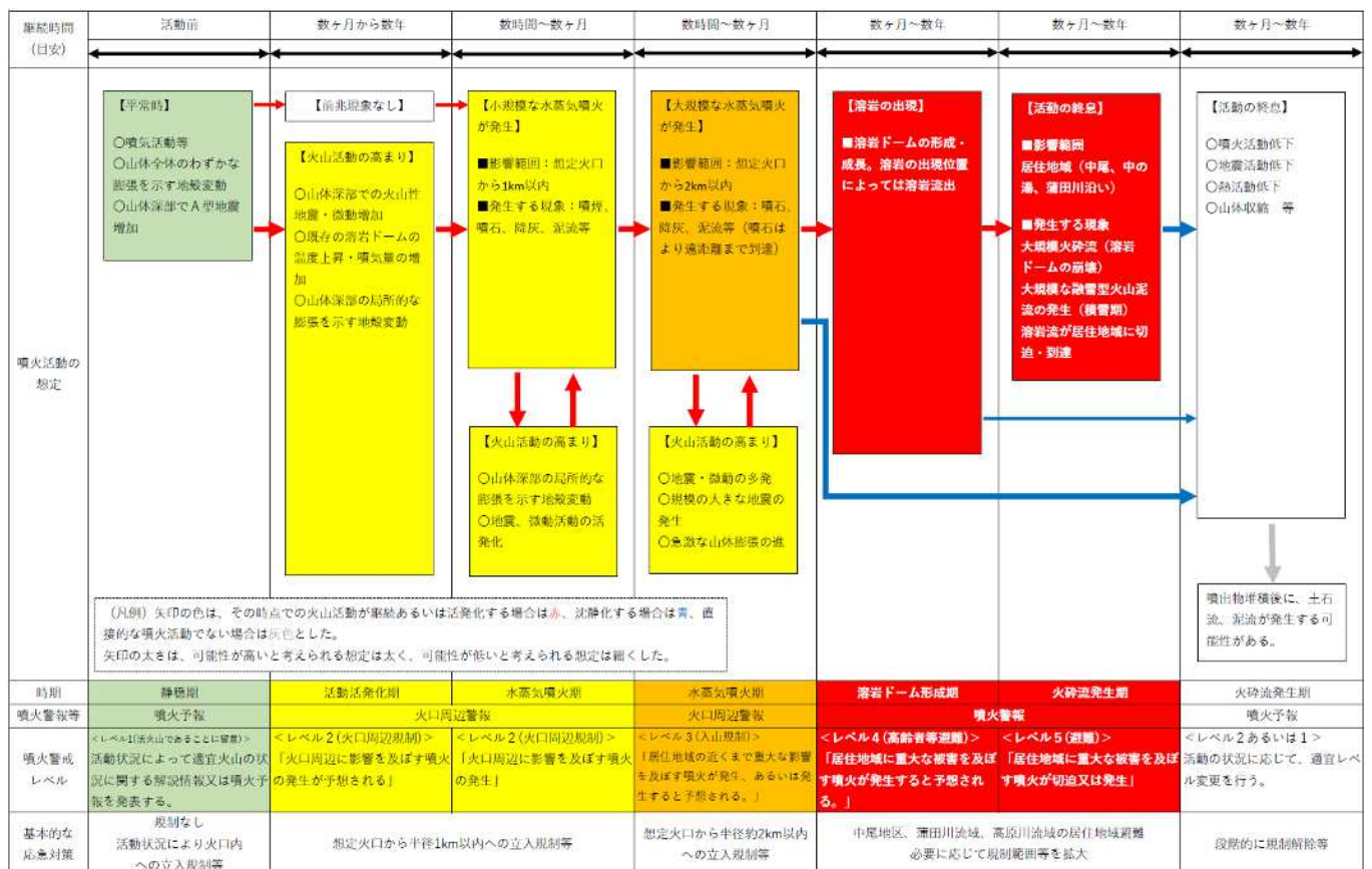
図-6-2 ケース 2 (マグマ噴火) の例
