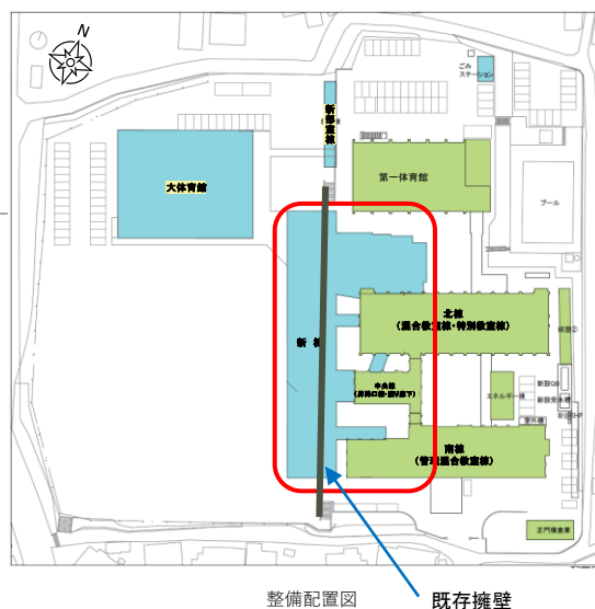
整備配置図
