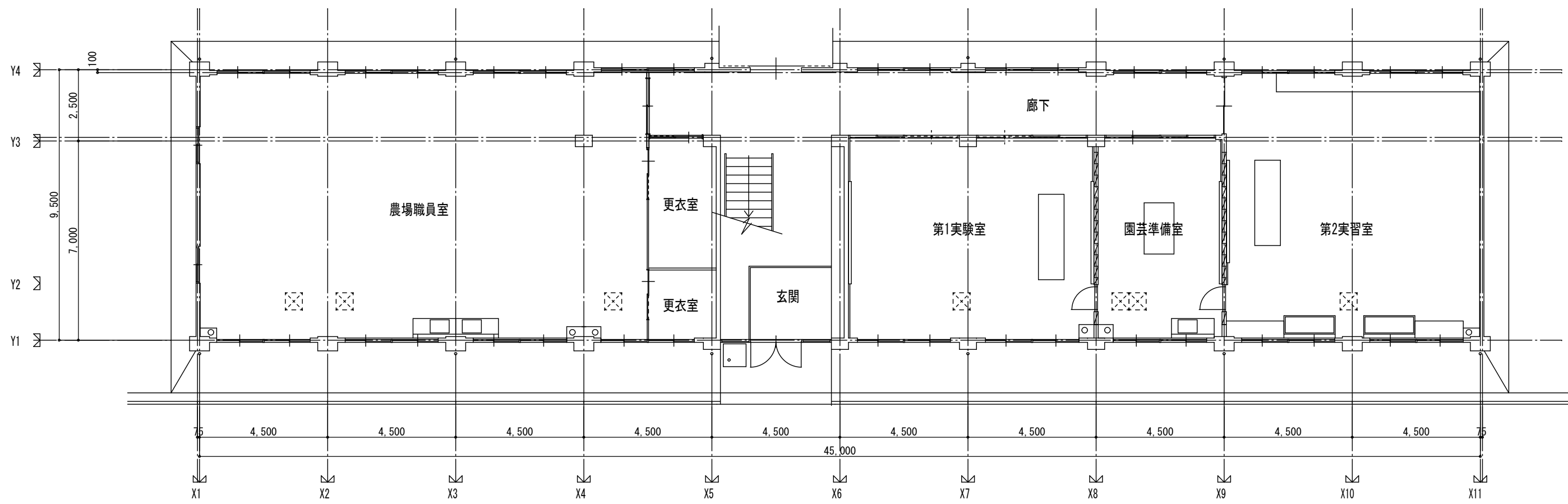
1階平面図
