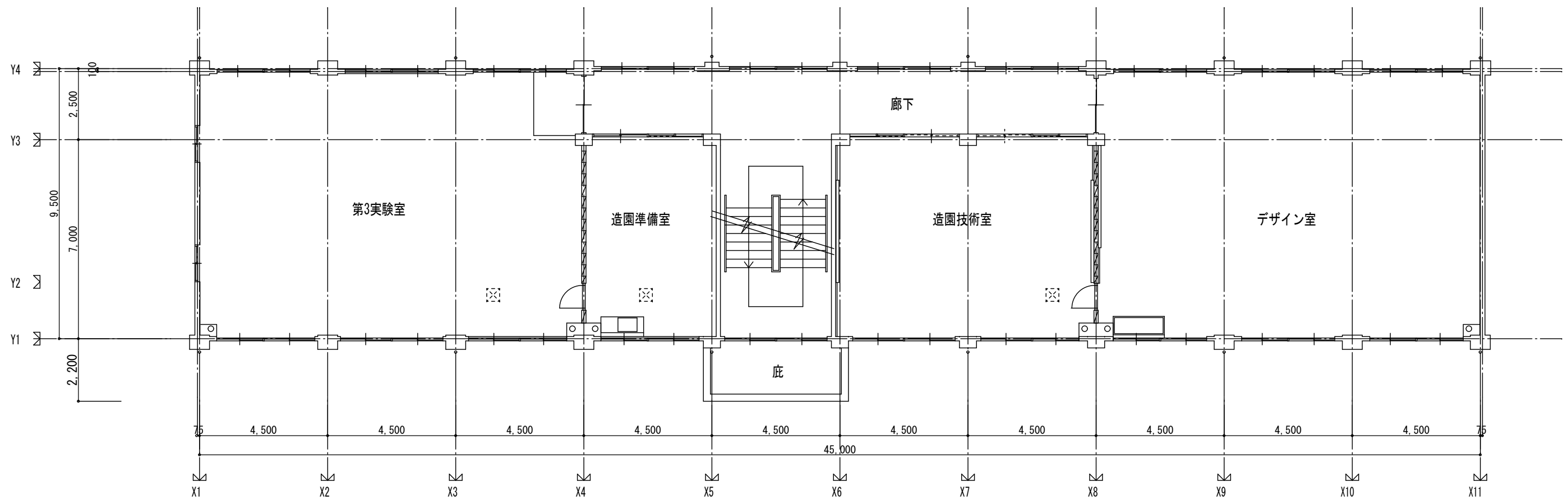
2階平面図
