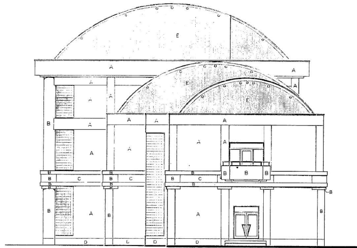
北立面图
