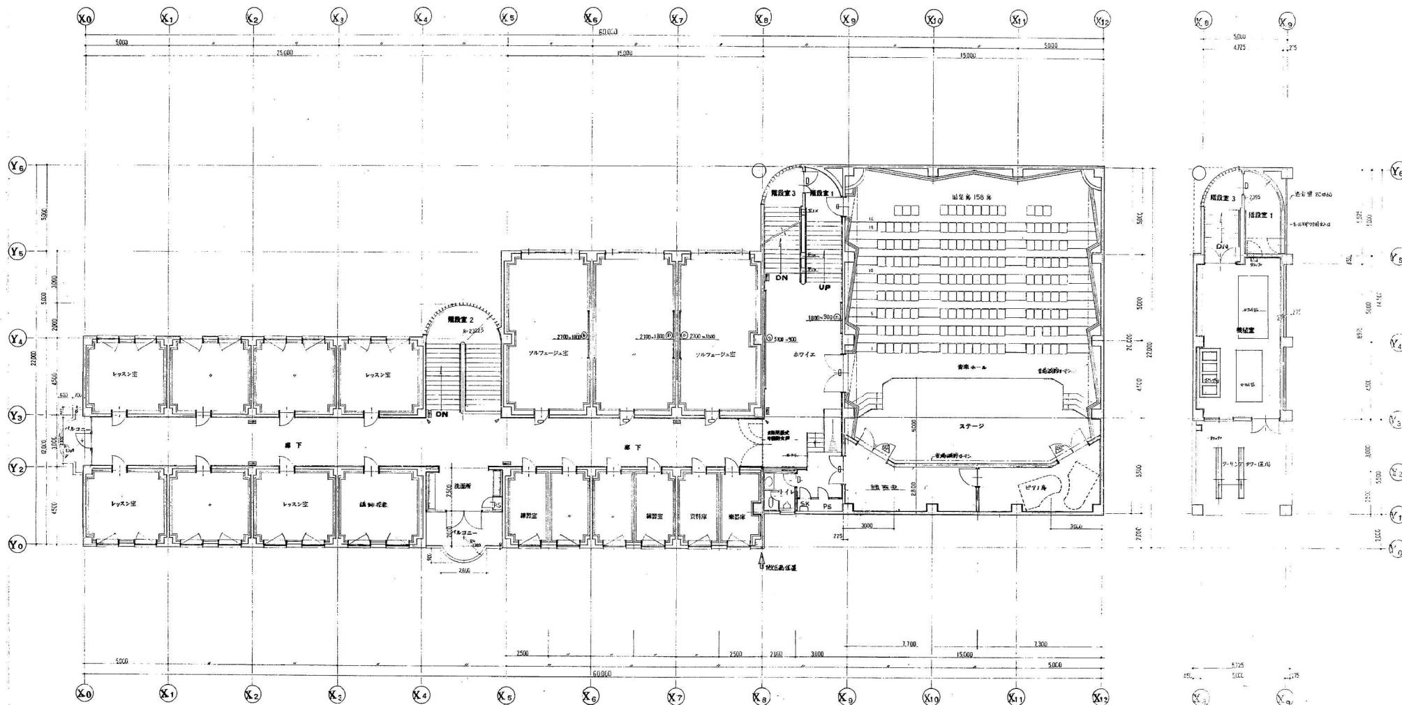
2階平面図
