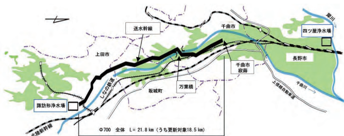
（参考）諏訪形浄水場～千曲市寂蒔 送水幹線概要図
