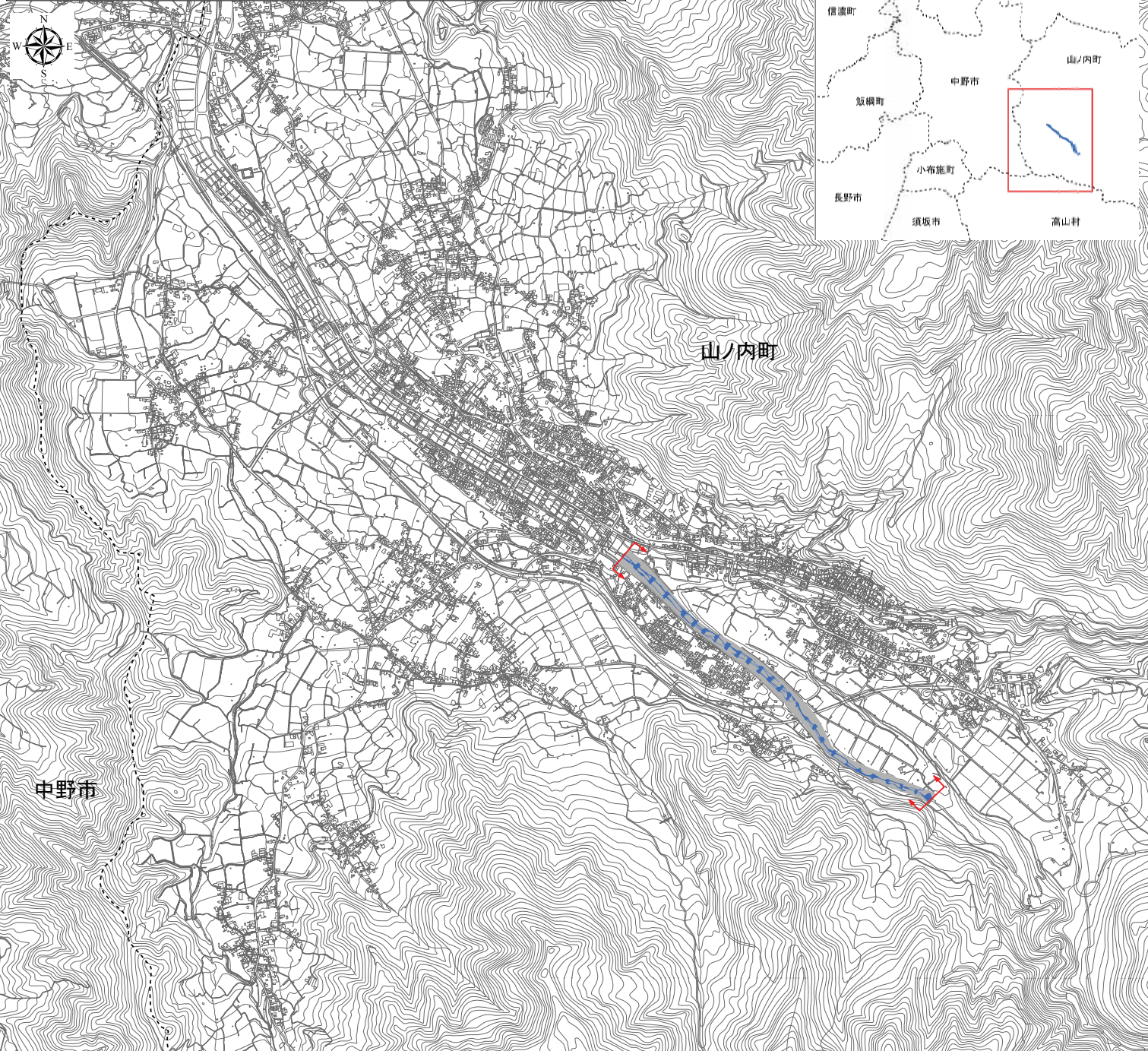
信濃川水系角間川 洪水浸水想定区域図 (計画規模降雨)
