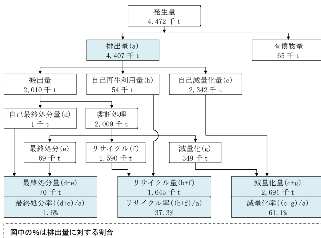
図 2-1-14 産業廃棄物の処理フロー (令和5年度)
