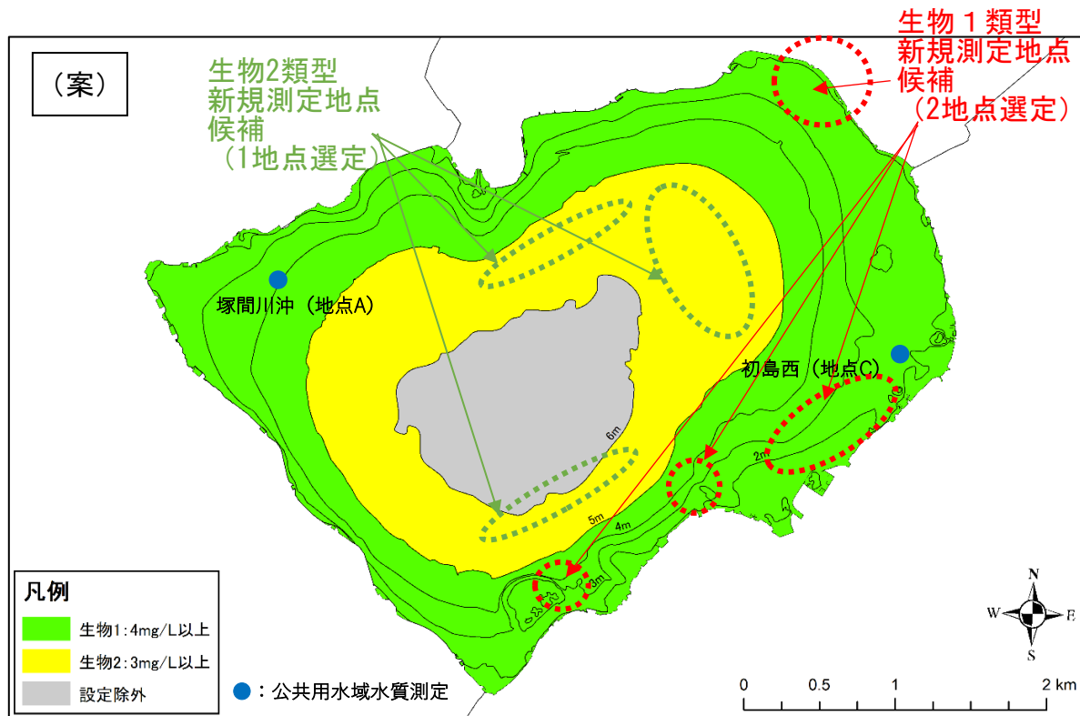
図－8 底層溶存酸素量の測定地点
