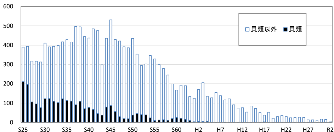
図－５ 諏訪湖における漁獲量の推移
