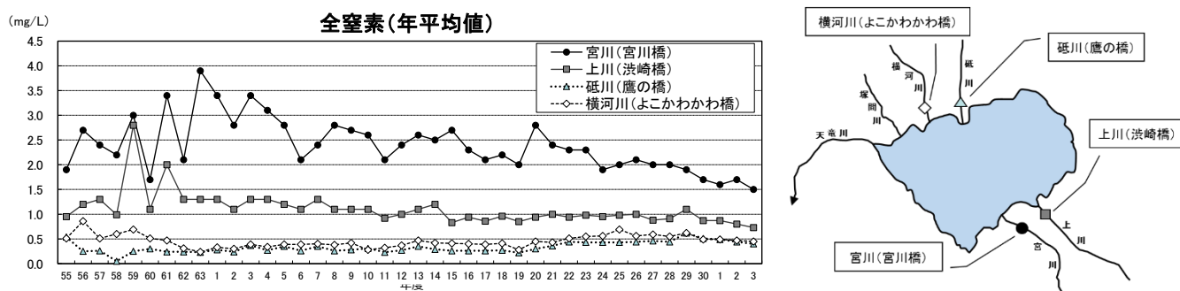
図-9 諏訪湖流入河川的全窒素の経年変化及び採水地点
