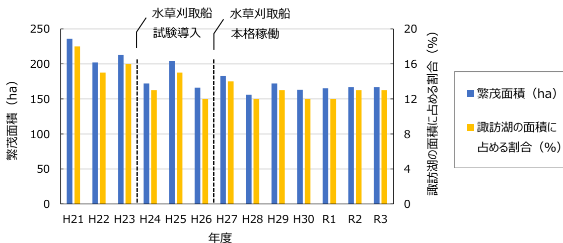
図－６ ヒシの繁茂面積の経年変化
