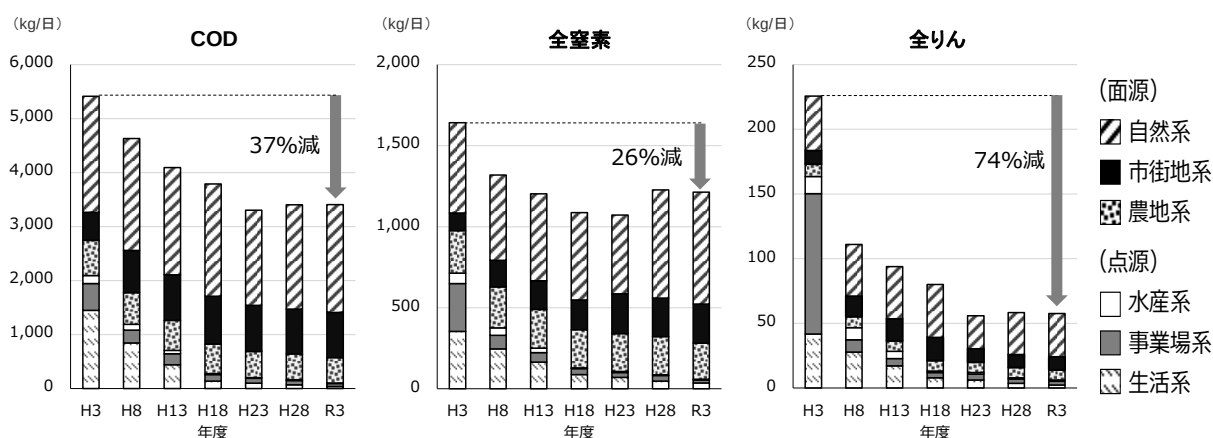
図－4 諏訪湖に流入する汚濁負荷量の推移
