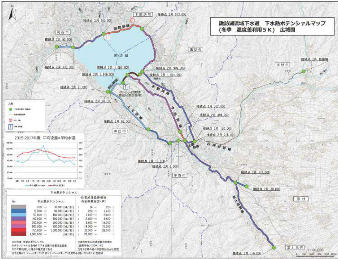
図表2-2-10 下水熱ポテンシャルマップ（諏訪湖流域下水道）
