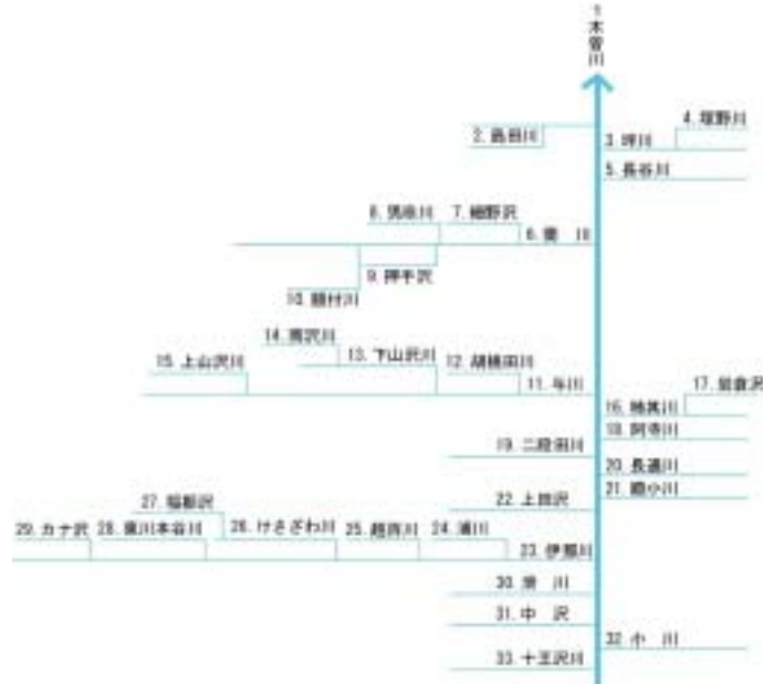
図 2.2.4 木曽川水系図
