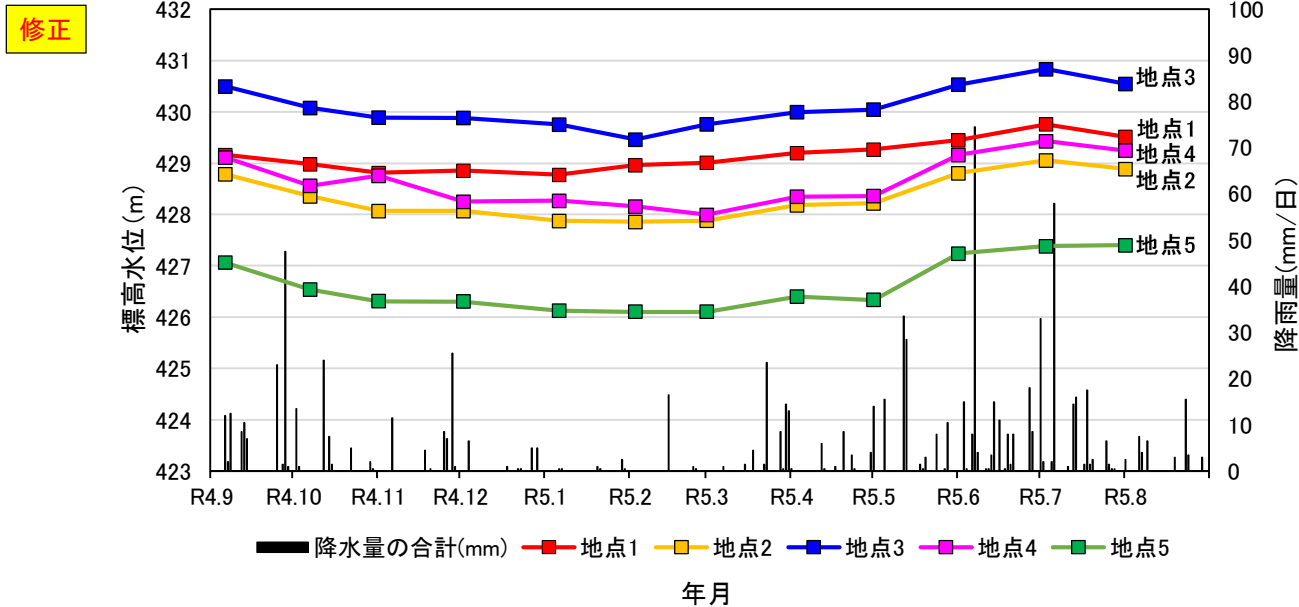
図 4.7-2 地下水位調査結果
