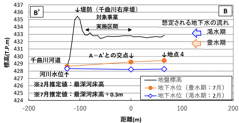
図 4.7-4 模式断面図
