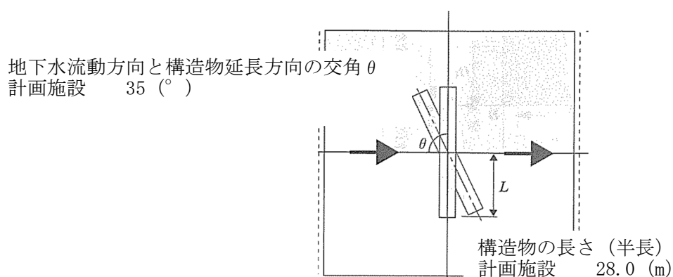
図 4.7-8 地下水影響の検討イメージ
