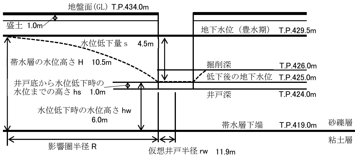
図 4.7-7 地下水影響の検討イメージ
