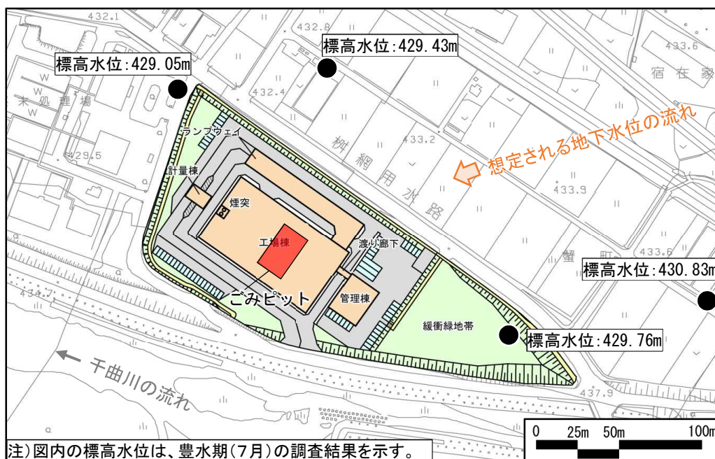
図 4.7-9 地下水の流れの方向とごみピットの位置
