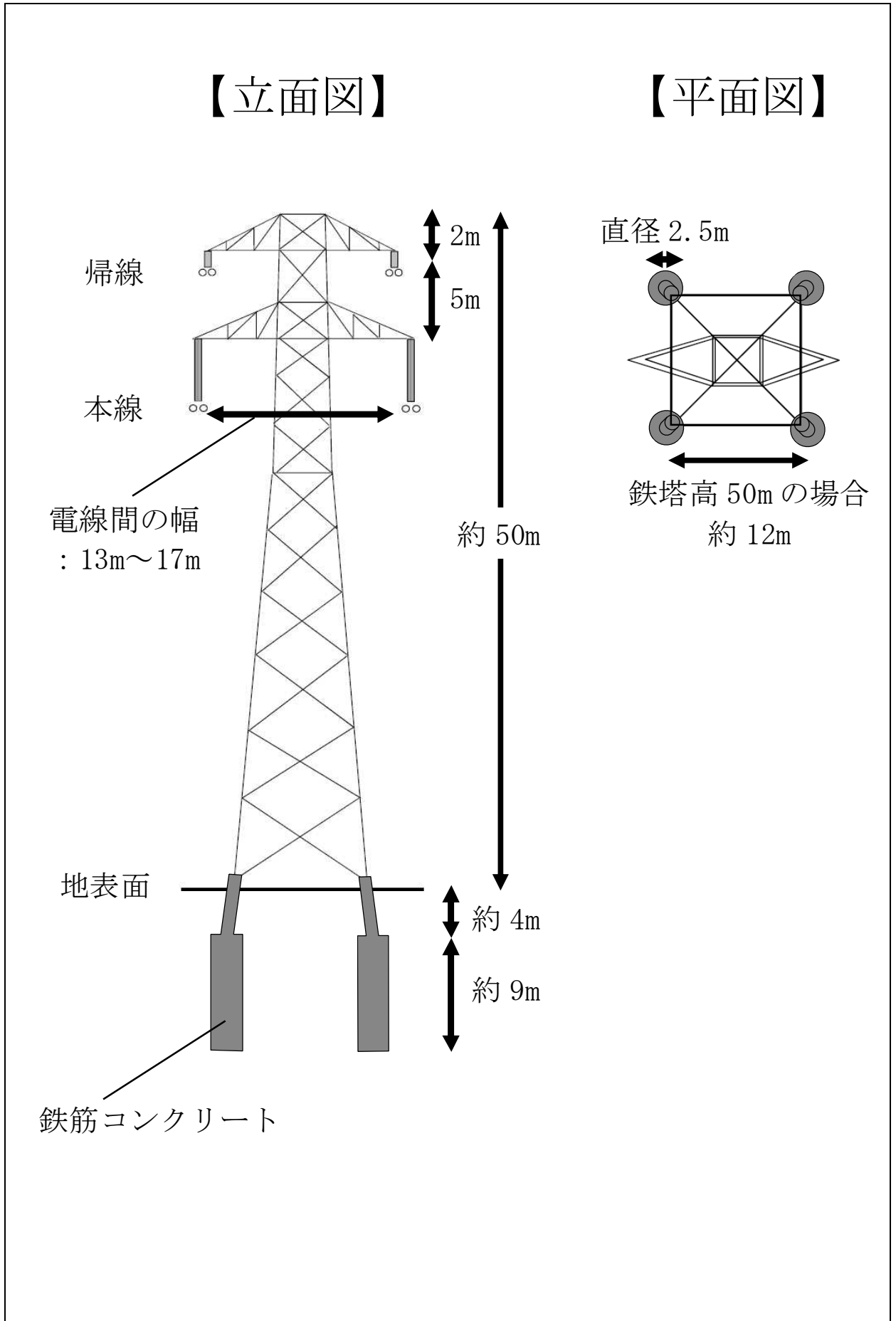
図 2. 2. 4-12 鉄塔形状図
