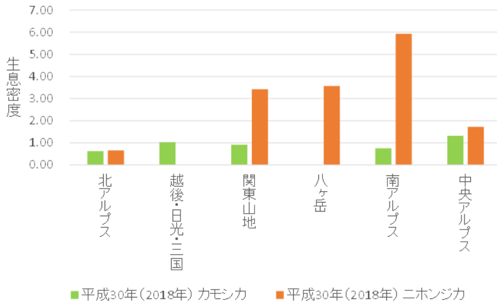
図7-5 各地域個体群のカモシカとニホンジカの生息密度 （区画法調査結果による）
