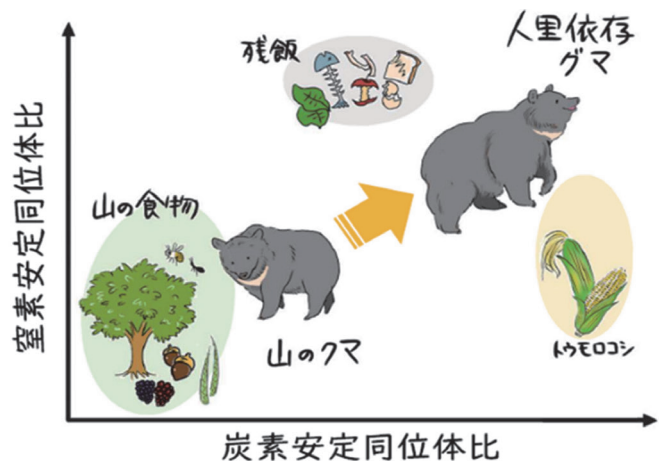
図1. 炭素・窒素安定同位体比によるツキノワグマの食性解析 山の食べ物を食べているクマ(の体毛の元素組成)は図の左下に分布する。人里に出没し農作物や残飯を食べているクマはこれらの元素組成に引っ張られて、図の上側や右側に分布する。
