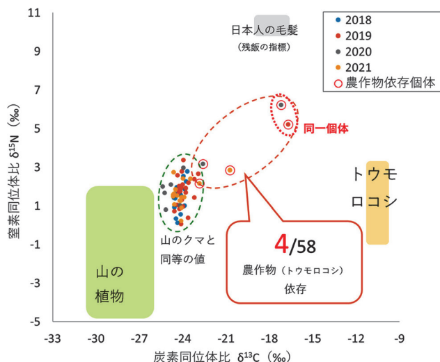
図2. 2018-21年に長野県伊那市周辺で錯誤捕獲されたツキノワグマの炭素・窒素安定同位体比
