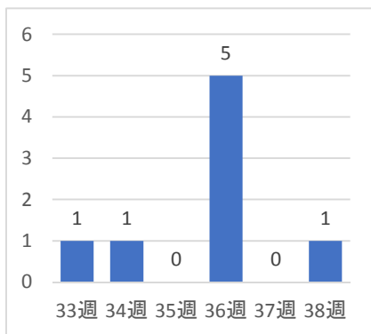
図1 週別発生状況(2018年、長野県)
