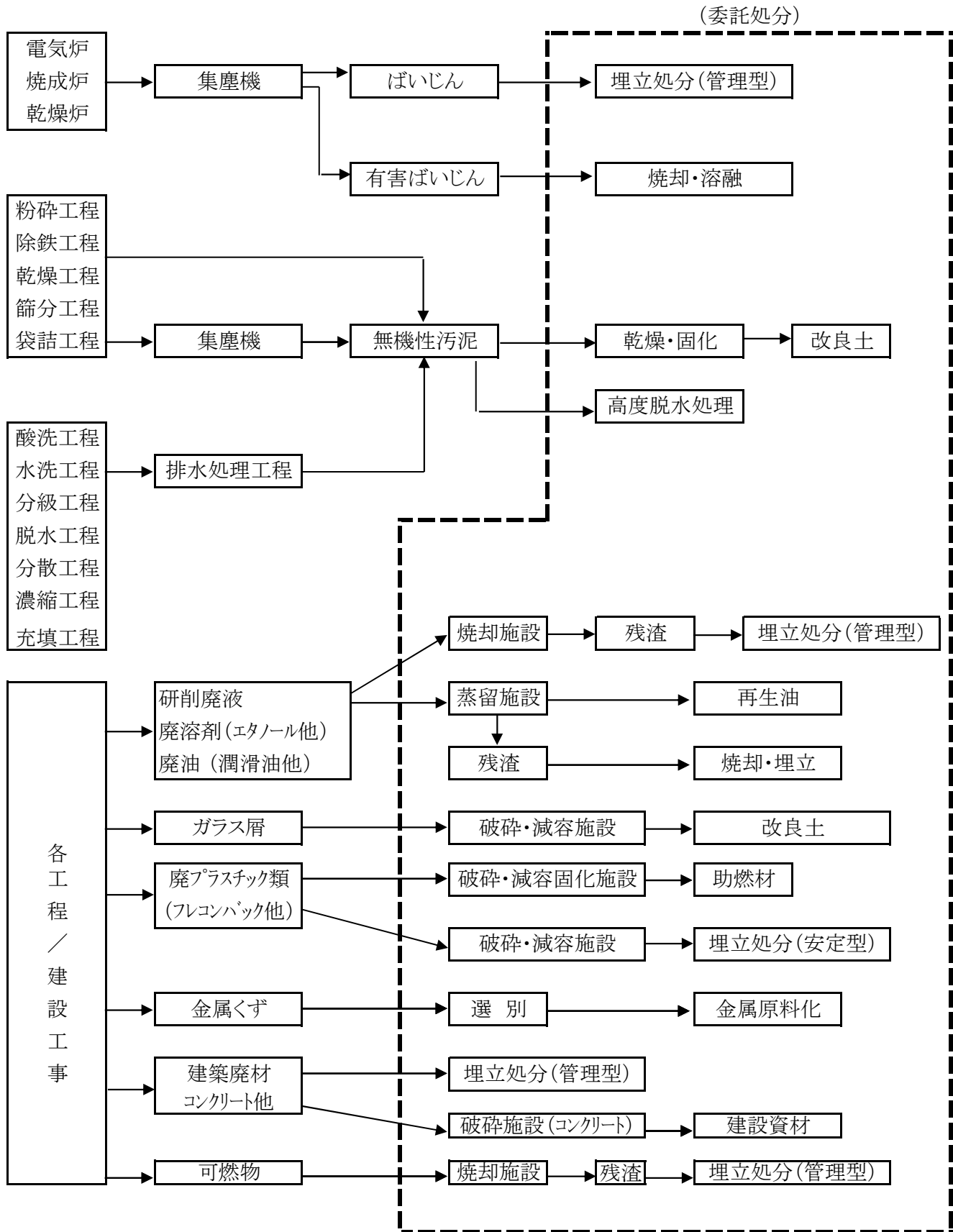
図4 廃棄物処理フローシート
