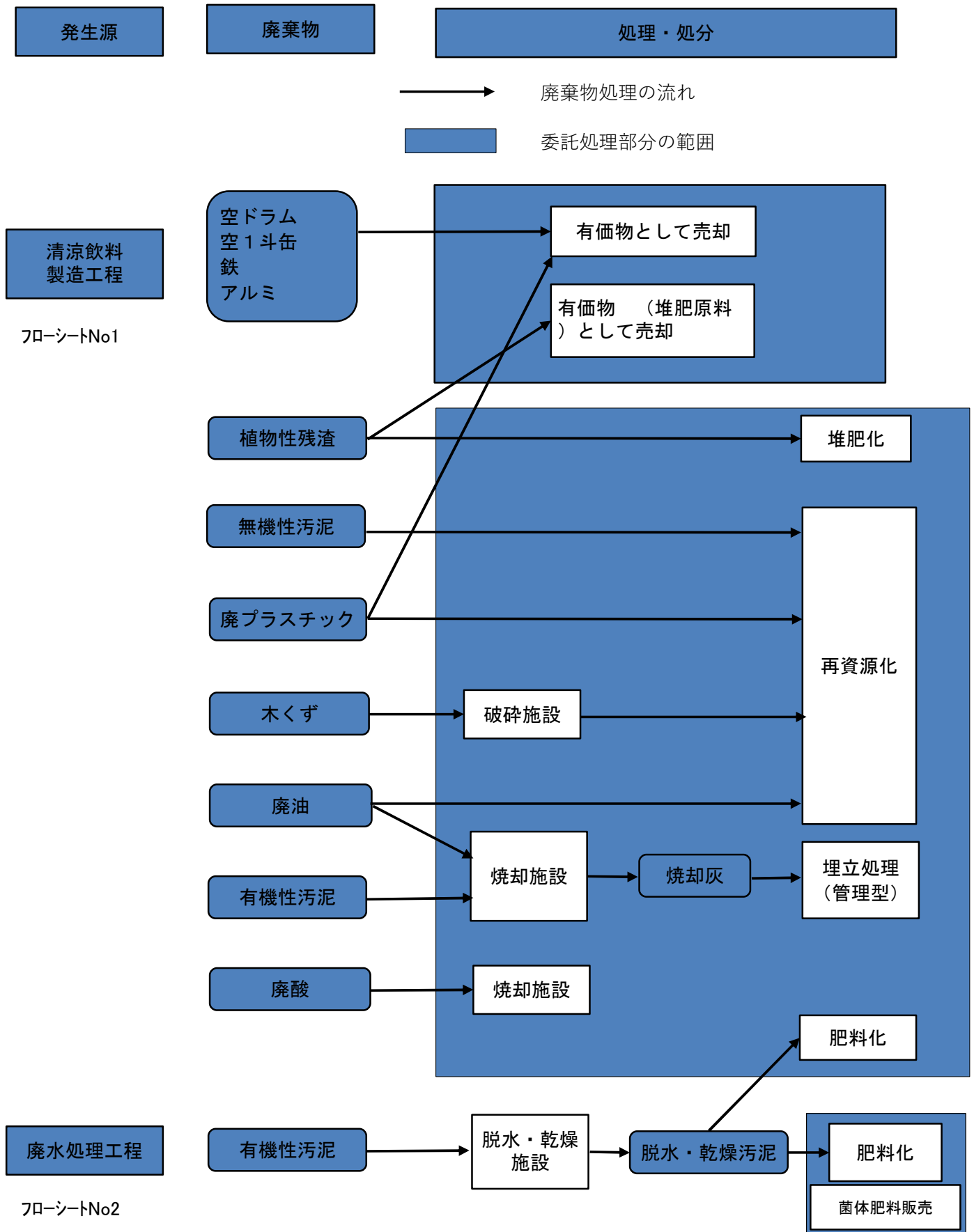
図3 廃棄物処理フロー図（現状）
