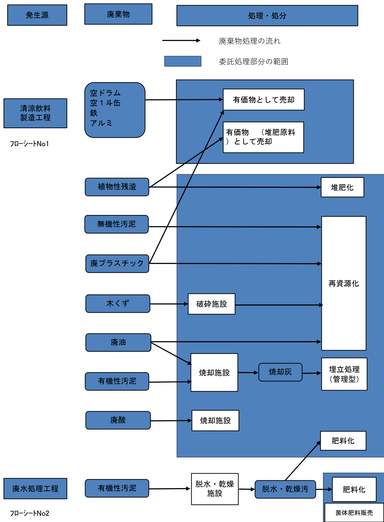
図3 廃棄物処理フロー図（現状）
