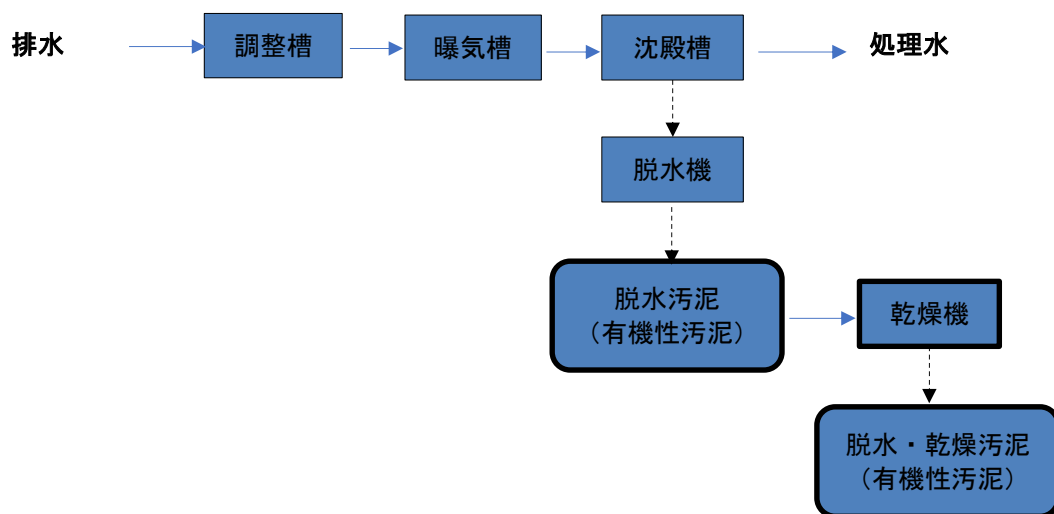
図2 廃水処理フローシート(NO.2)
