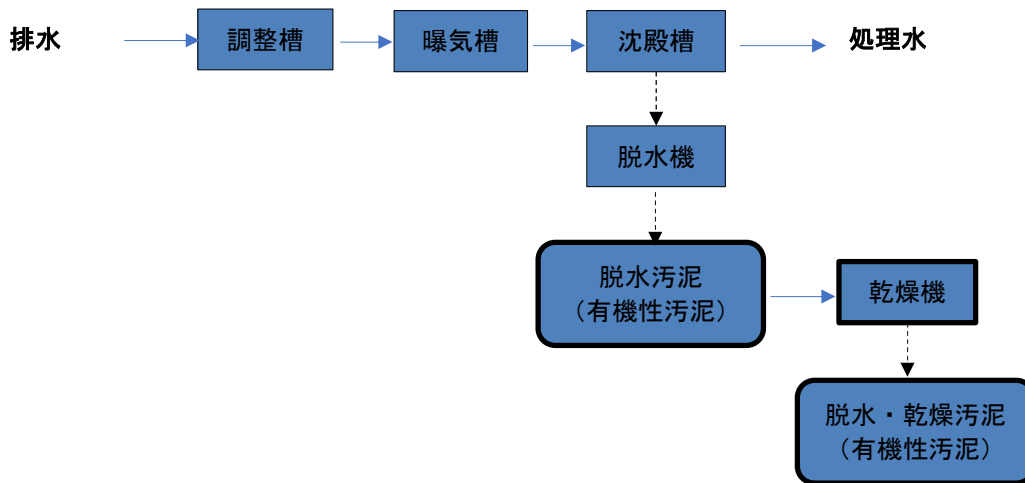
図2 廃水処理フローシート(NO.2)
