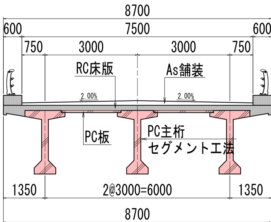
ポステン方式単純コンポ橋：標準断面図
