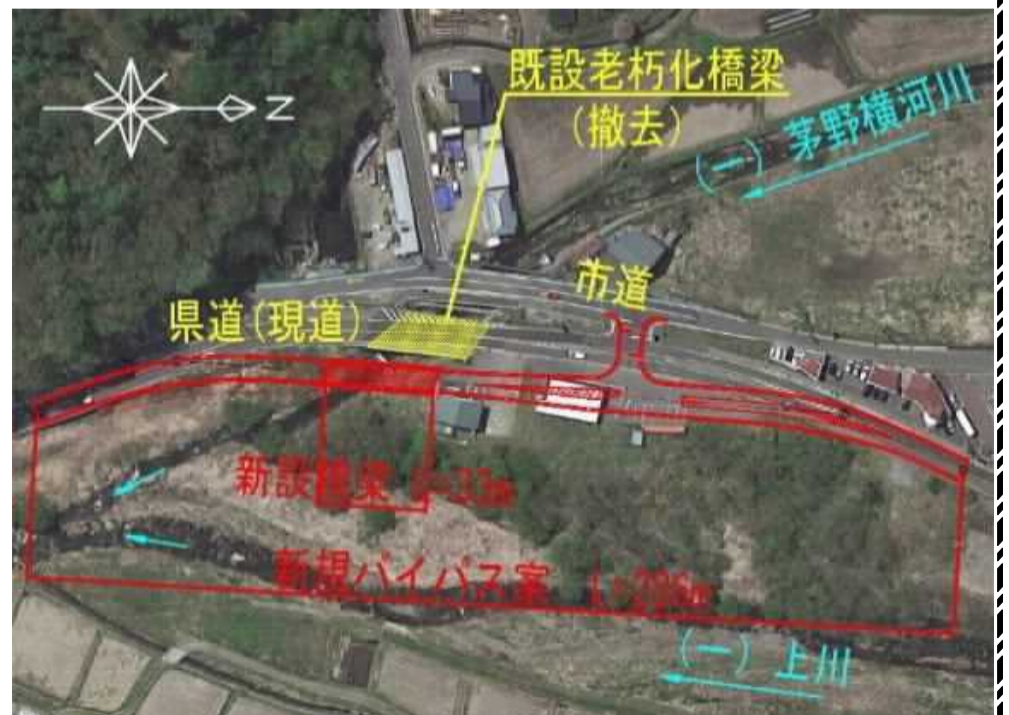
【全体平面図】
