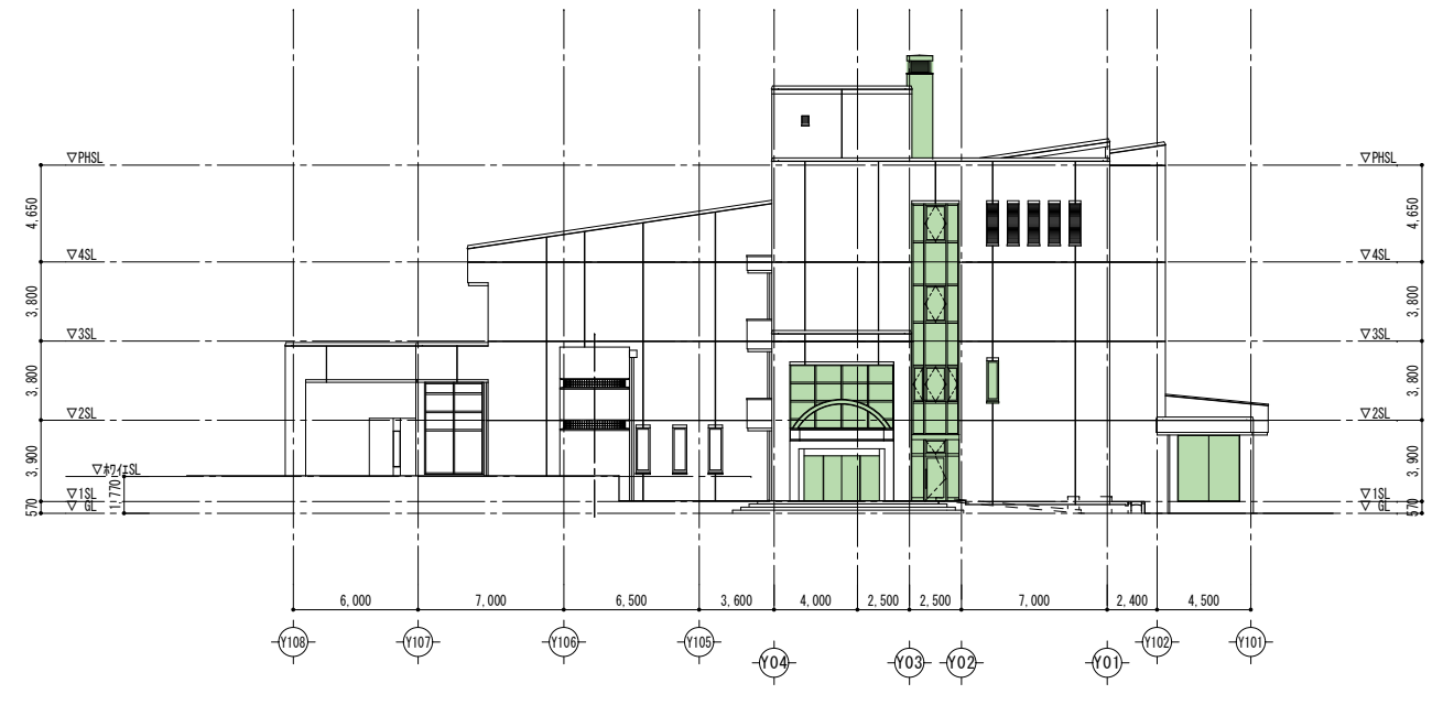
西側立面図 S=1/200
