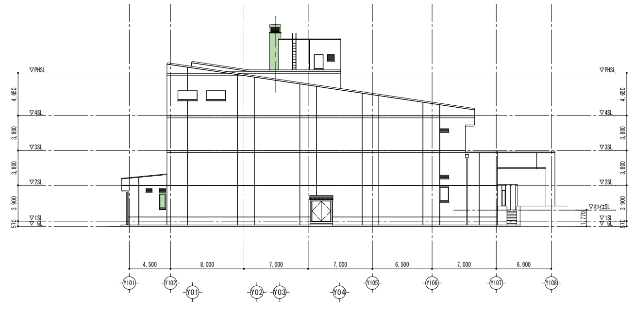
東側立面図 S=1/200
