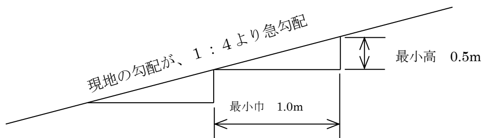
図1-3-1 盛土基礎地盤の段切
