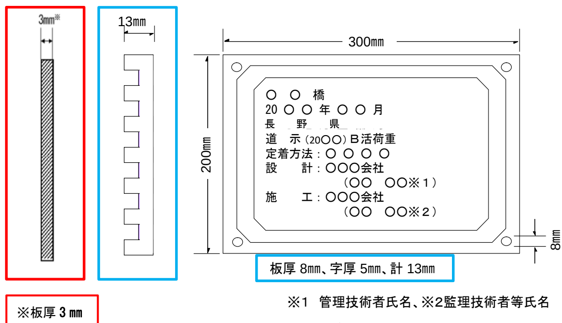
図 1-2-2：銘板の寸法及び記載事項
