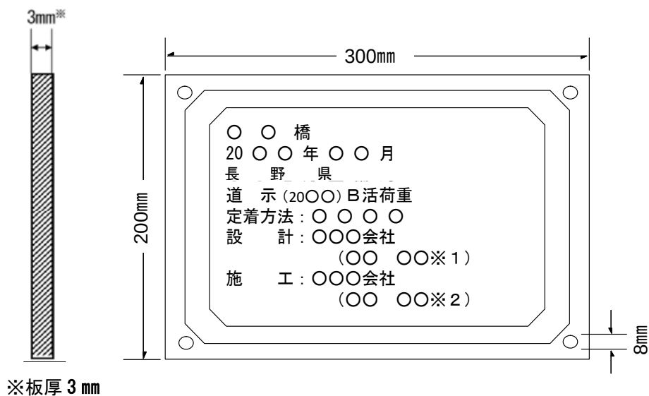
図 1-2-2：銘板の寸法及び記載事項
