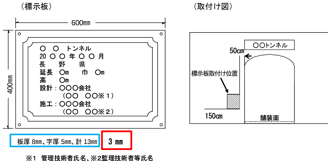
図 6-6-2 標示板の設置イメージ図
